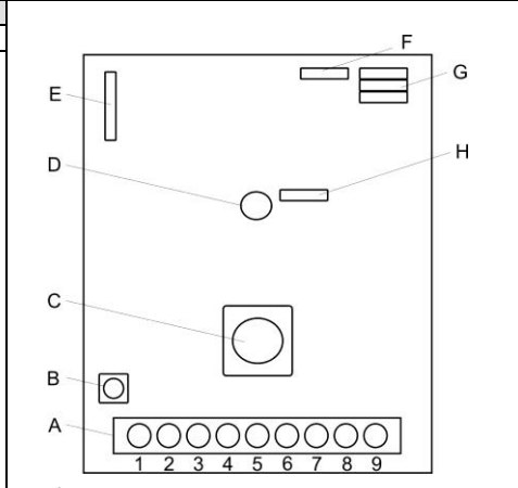
Fig. 2: A: Bornes de raccordements/ Terminale di connessione B: Contact autoprotection/ Contatto antisabotaggio C: Composent PIR dual/ Sensore PIR D: DEL/LED E: pont enfichable de mémoire/ Ponticello memoria F: Pont enfichable du test de fonctionnement/ Ponticello per walk-test G: Pont enfichable du compteur d'impulsion/ Contatore d'impulsi H: Pont enfichable de la DEL/ Ponticello LED Bornes de raccordements/ Terminale di connessione 1 Mémoire/ Memoria 2 Test de fonctionnement/ Walk-Test 3&4 Autoprotection/ Manomissione 5 libre/ Libro 6&7 Alarme/ Allarme 8&9 Tension d'alimentation/Ingresso tensione (GND, +12V)
