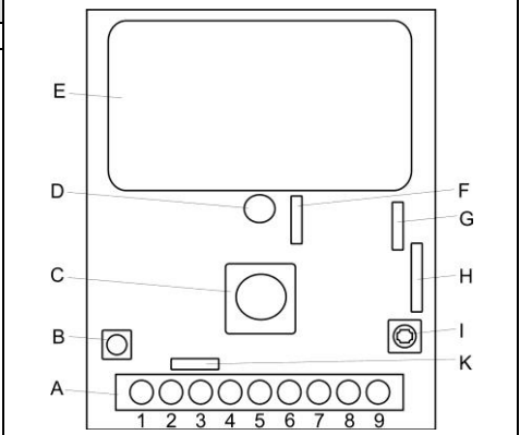
Fig. 1 A: Bornes de raccordements/ Terminale di connesse B: Contacte autoprotection/ Contatto antisabotaggio C: Composent PIR dual/ sensore PIR duale D: DEL/LED E: Doppler Module/ modulo doppler F: Pont enfichable de la DEL/ ponticello LED G: Pont enfichable du compteur d'impulsion/ Ponticello contatore di impulsu H: pont enfichable de mémoire/ ponticello memoria I: Potentiomètre micro-ondes/ Potenziometro MW K: Pont enfichable du test de fonctionnement/ ponticello per walk-test
