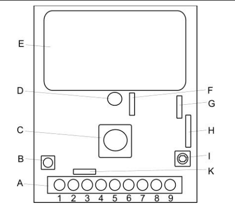
Fig. 1 A: Aansluitklemmen/ TiJslutningsliste B: Tamper-contacten/Sabotagekontakt C: dual PIR element/ dual PIR-element D: LED E: Doppler Module/ Doppler-Modul F: geleiderbrug LED/ LED-jumper G: geleiderbrug impulssteller/ Jumper impulssteller H: geleiderbrug geheugen/ Jumper til hukommelse I: potentiometer radar/ Potentiometer MW K: geleiderbrug looptest/ Jumper GA-TEST Aansluitklemmen/ TiJslutningsliste 1 geheugen/ Hukommelse 2 loop-test/ GÅ-test 3&4 Tamper/ Sabotage 5 vrij/Fri 6&7 alarm 8&9 spanningstoevoer/ Spændingsindgang (GND, +12V)
